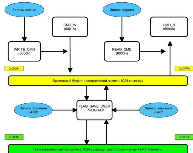
Рис.8. Блок-схема процедур чтения и записи пользовательской программы.
