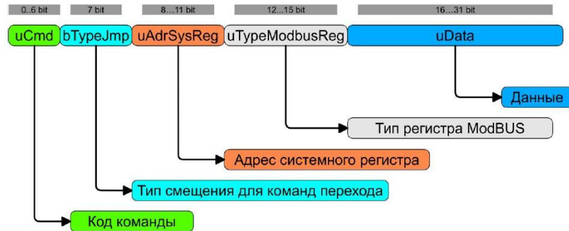
Рис.9 – структура инструкции пользовательской программы
