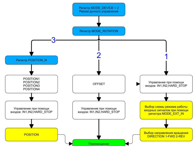
Рис.7. Блок-схема выбора режима работы при управлении приводом внешними сигналами
