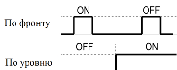
Рис.5. Диаграмма управляющих сигналов START/STOP и DIR.
