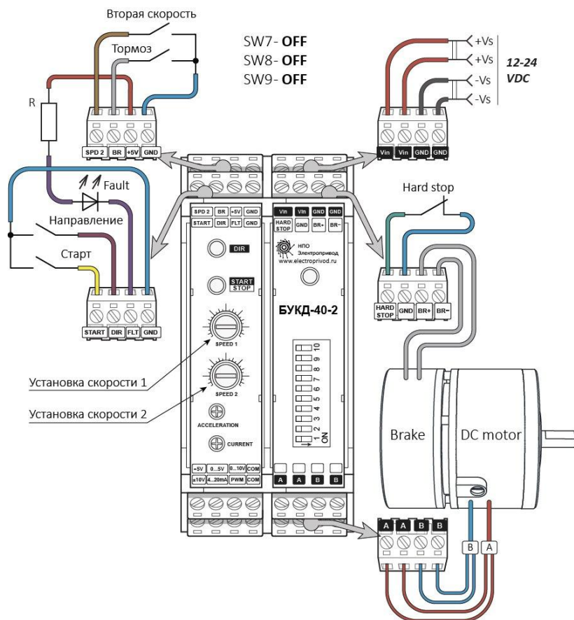
Рис.3. Схема подключения при управлении от встроенного потенциометра
