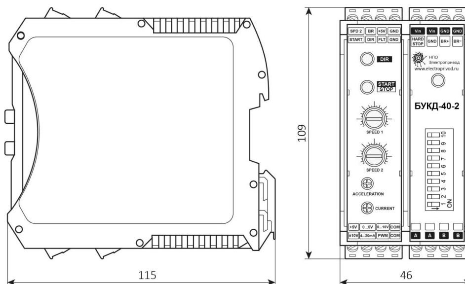
Рис.1 Размеры контроллера БУКД-40К-2
