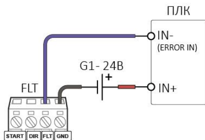
Рис. 7. Пример подключения к внешнему ПЛК.
