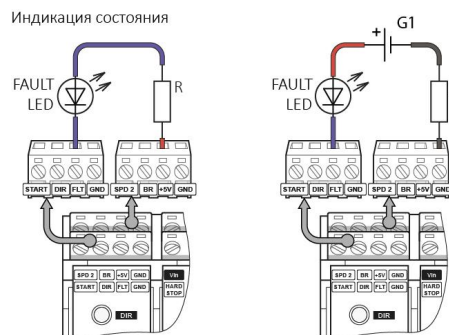
Рис. 8. Примеры подключения светодиода индикации.
