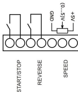
Рис. 3. Подключение управляющих
