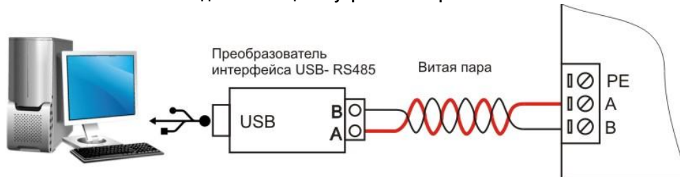
Рис. 4. Схема подключения по шине RS-485.
