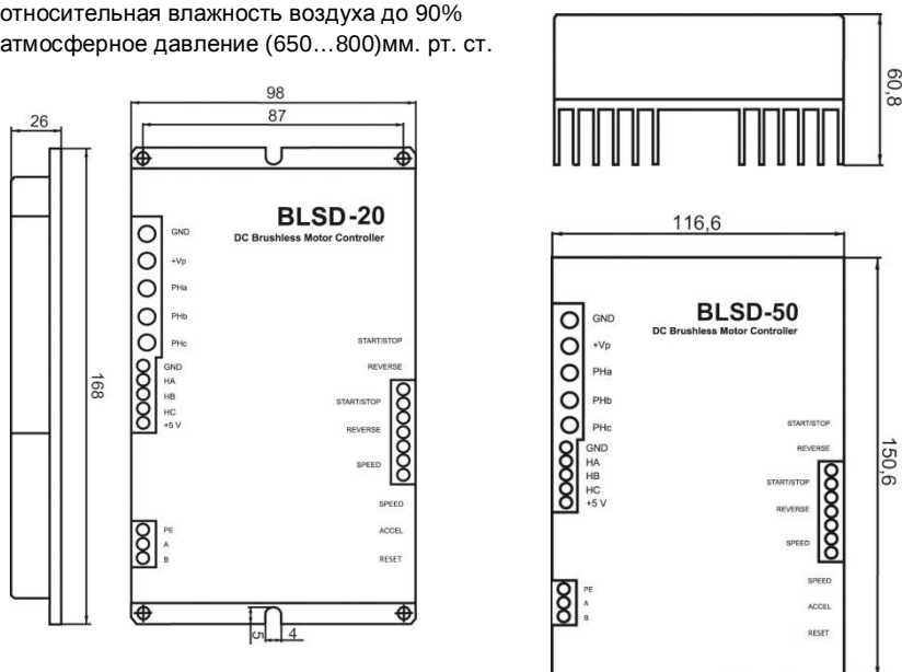
Рис. 1. Габаритные и присоединительные размеры блока BLSD
