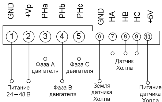
Рис. 2. Схема подключения
