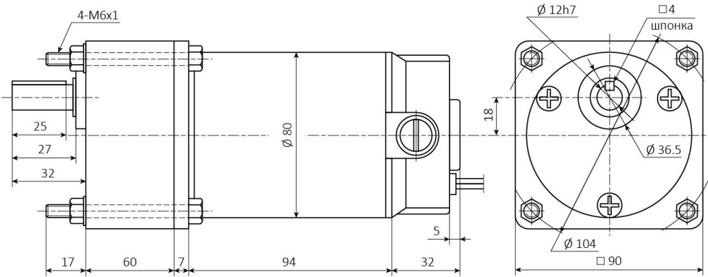
Габаритные и присоединительные размеры мотор-редуктора SF7152
