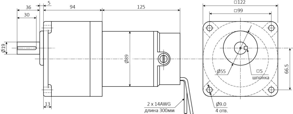
Габаритные и присоединительные размеры мотор-редуктора SF8156
