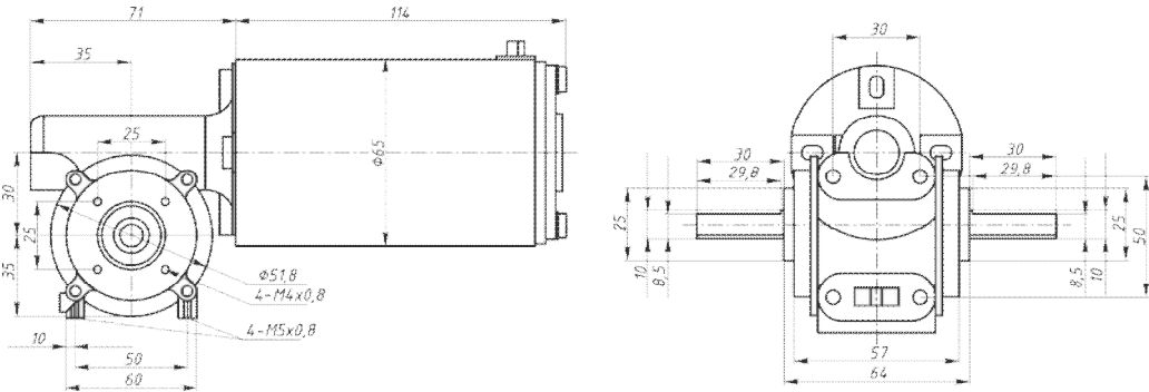
Габаритные и присоединительные размеры мотор-редуктора WG5946
