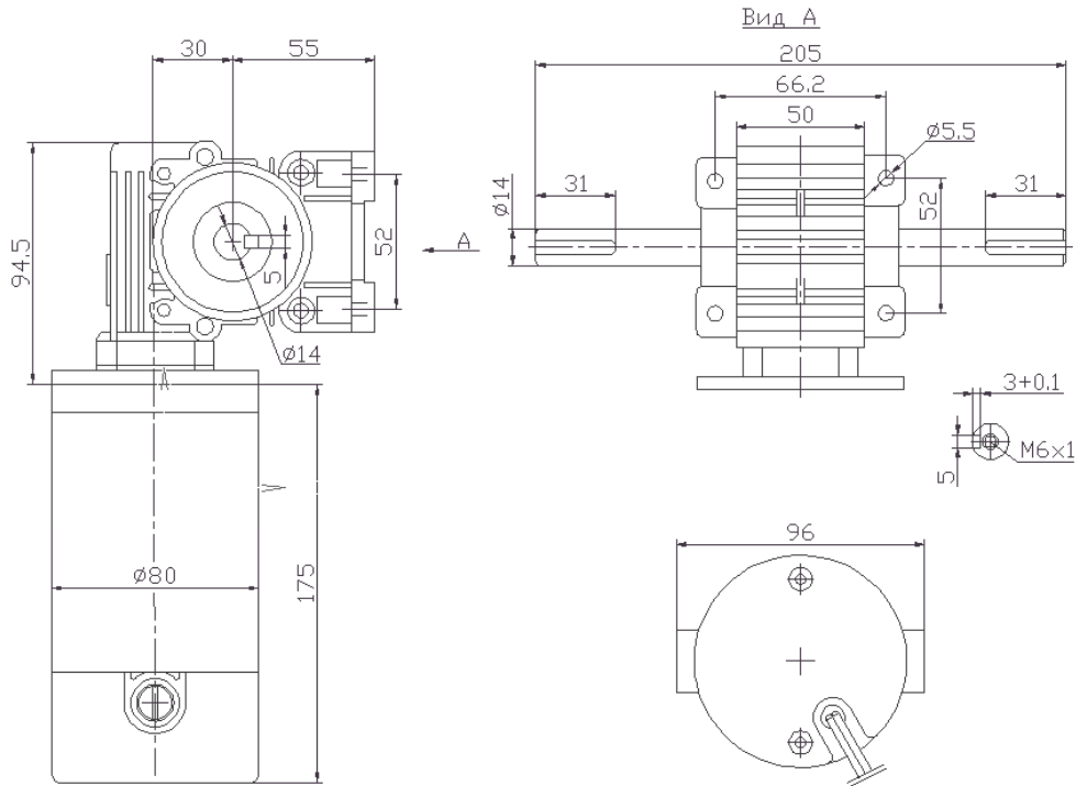
Габаритные и присоединительные размеры мотор-редуктора WG7185
