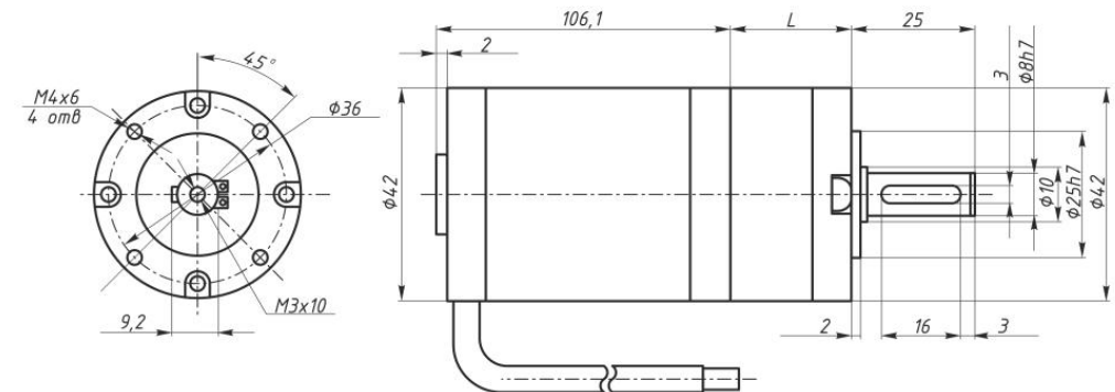
Рисунок 1. Габаритные и присоединительные размеры МРК-42
