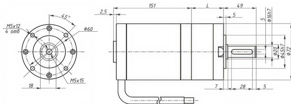
Рисунок 4. Габаритные и присоединительные размеры МРК-72
