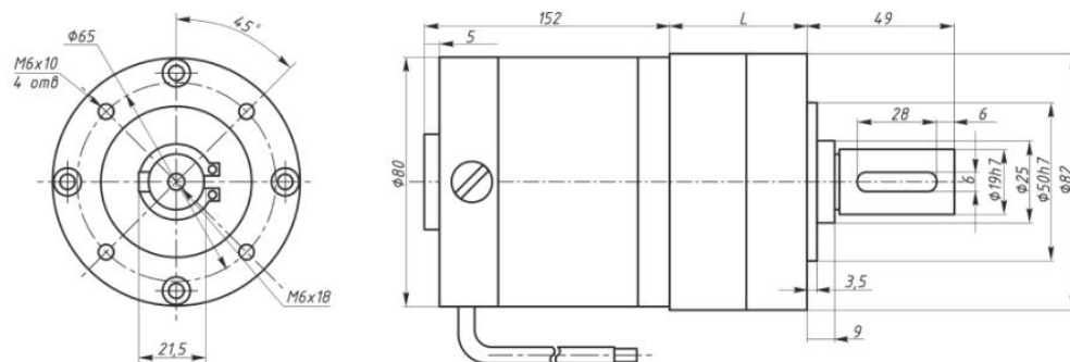
Рисунок 5. Габаритные и присоединительные размеры МРК-82
