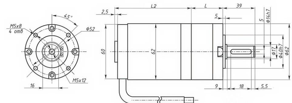
Рисунок 3. Габаритные и присоединительные размеры МРК-62
