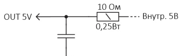
Рис. 10. Аналоговый выход 5В
