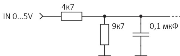
Рис. 7. Аналоговый вход 0...5В
