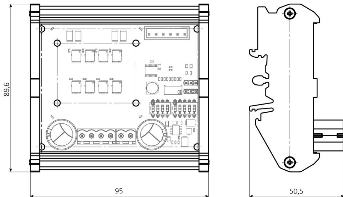
Рис. 5. Габаритные и присоединительные размеры БУШД-4.2Ф и БУШД-8.0
