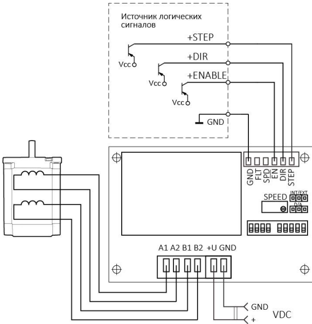
Рис. 2а. Схема подключения драйвера серии БУШД в режиме управления логическими сигналами STEP/DIR/EN
