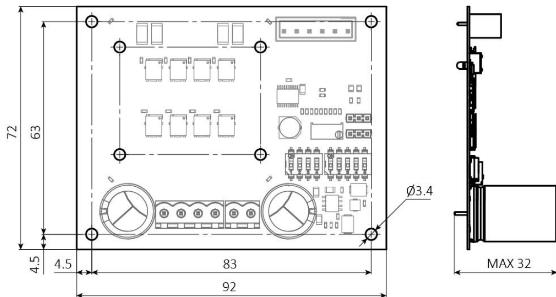
Рис. 4. Габаритные и присоединительные размеры БУШД-4.2 и БУШД-8.0
