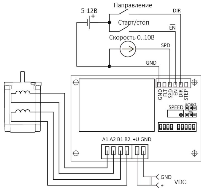
Рис. 2б. Схема подключения драйвера серии БУШД в режиме управления аналоговым сигналом 0 - 10 В
